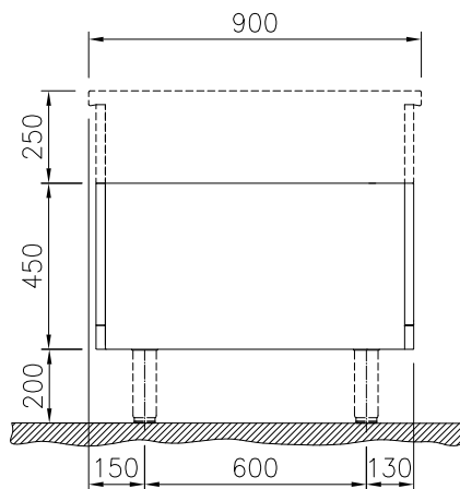
Boven aanzicht
